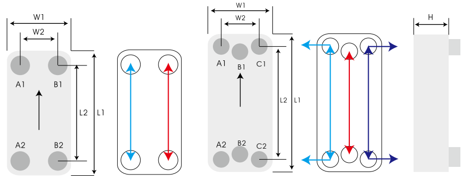
K215D/K415D: 二回路 -6 穴タイプ
