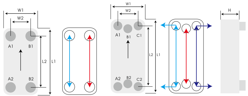
B236D/B415D/B416D: 二回路 -6 穴タイプ
